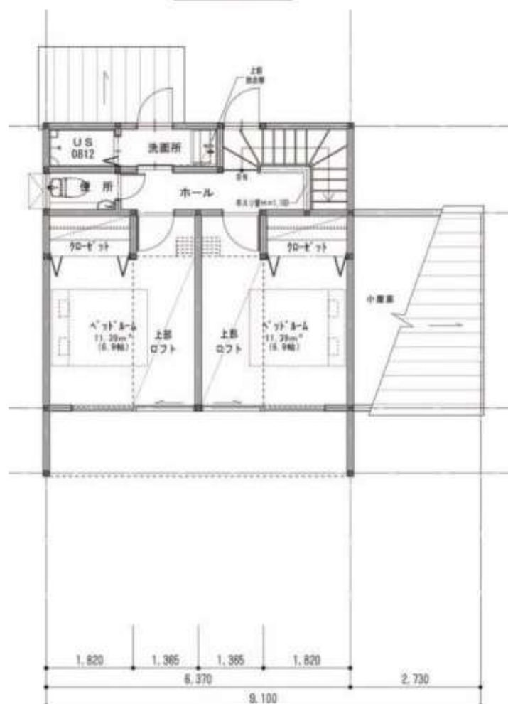
1 階平面図
