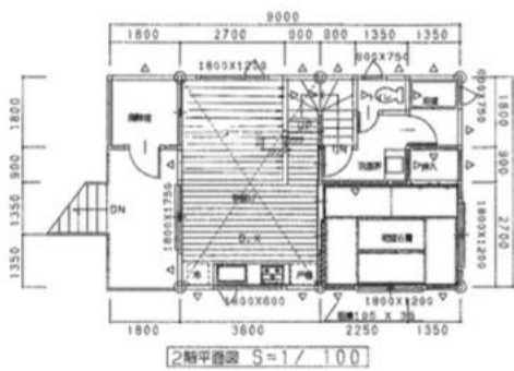
2階平面図 S=1/100
