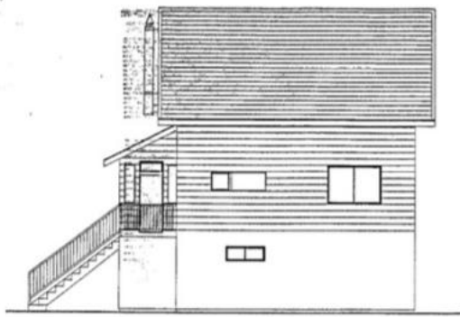
南東立面図 S=1/100
