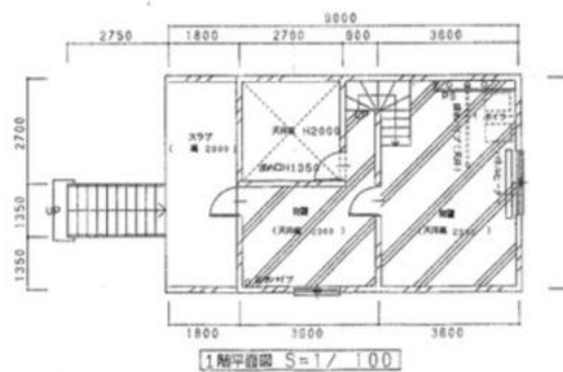
1階平面図 S=1/100
