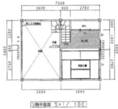
3階平面図 S=1/100
