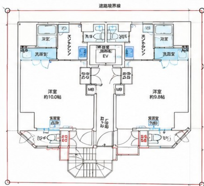
3～8階平面図
