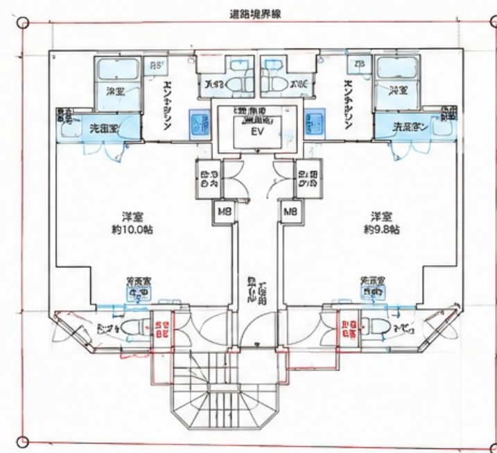
2階平面図
