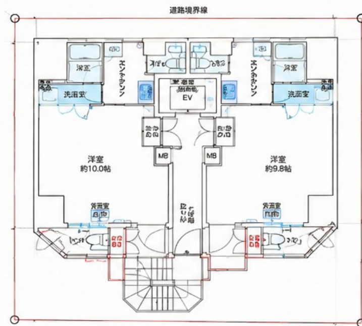
9階平面図
