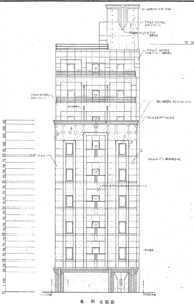
北側立面図
