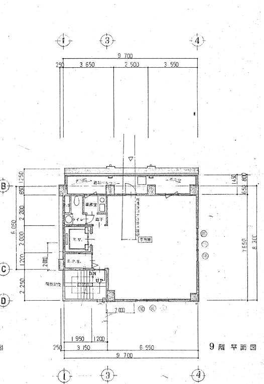
8階平面図
