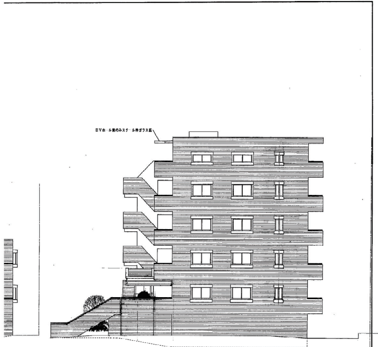
西側立面図 1/100
